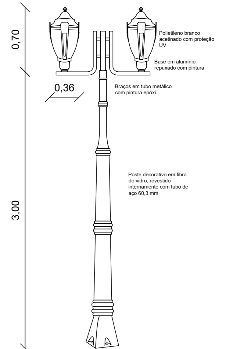
2 DETALHAMENTO - POSTE DECORATIVO Escala: 1:25
